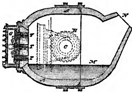
FIG. 2.—Bessemer Converter.
